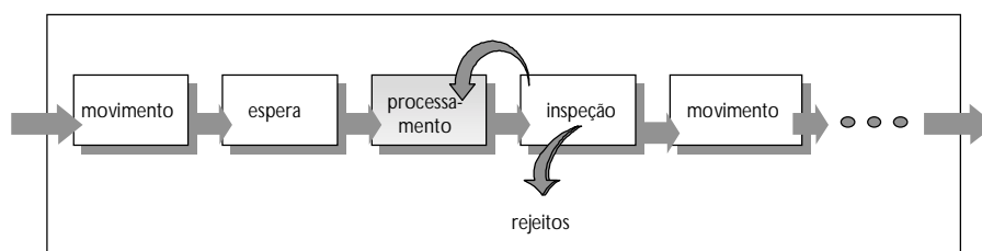
Figura A.1: Representação do processo de produção segundo Koskela (1992)
